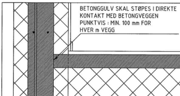
Detalj 1 - 206-3 - 1:10
