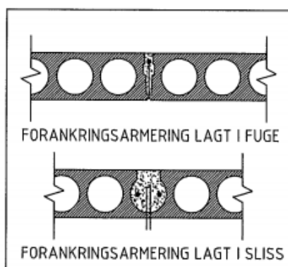
Detalj 2 - 204-3 - 1:20
