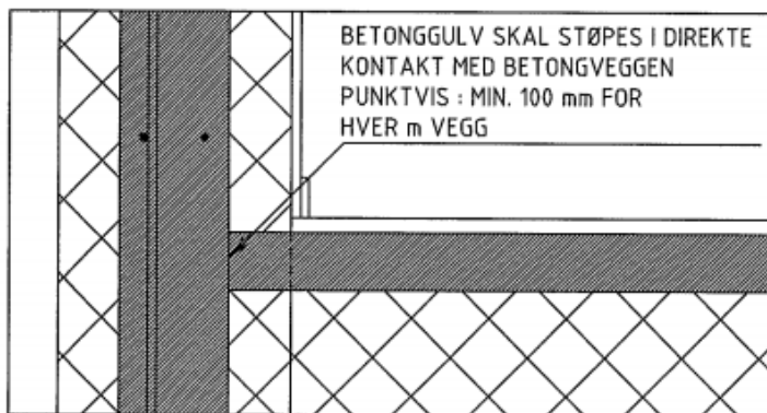
Detalj 1 - 204-3 - 1:10
