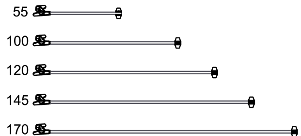
Lengder støttestag / Lengths support brace
